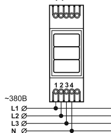
Схема подключения
