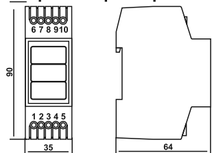
Габаритные размеры
