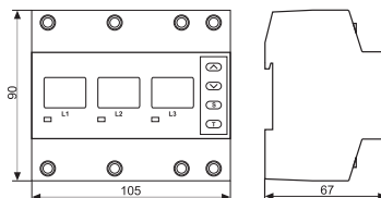
Рис.2. Габаритные размеры
